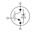
X027a SOT-227B (miniBLOC)
