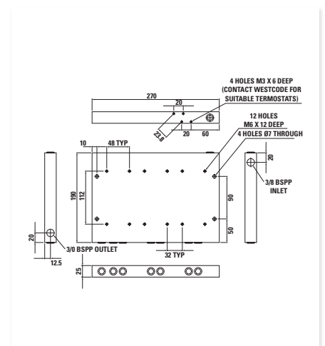
WCL9 - WS65 COOLER
