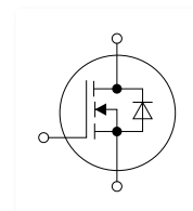
X011b TO-263AB
